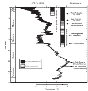
F1. Cenozoic \delta^{18}\text{O} data, p. 10.
